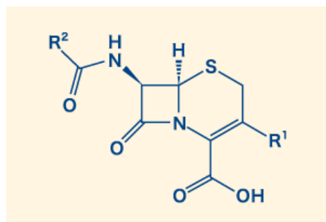
図2: セフェム系の構造式
